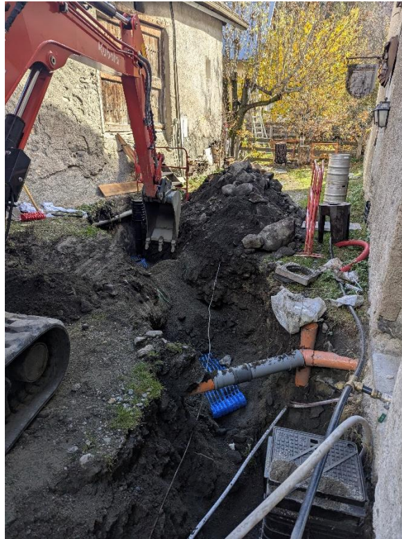
Figure 2 : Branchement neuf MME CLATOT
